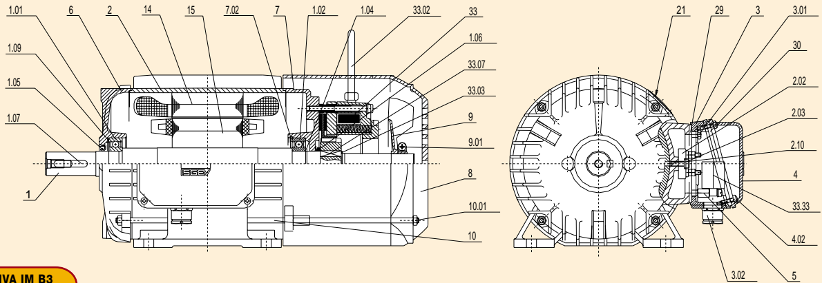
FORMA COSTRUTTIVA IM B3 ASSEMBLY IM B3
